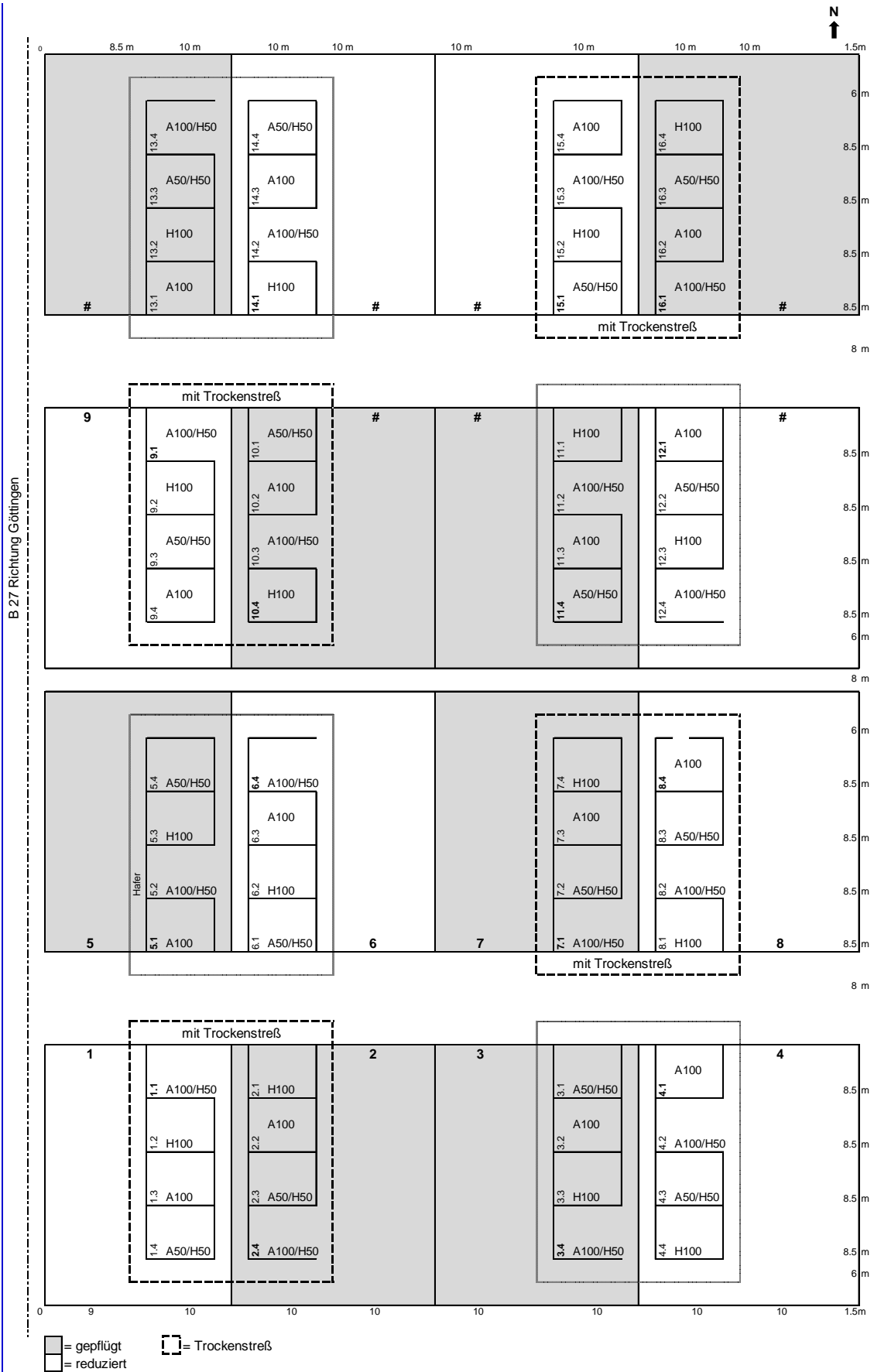
Feldplan: Vertikale Wurzelverteilung in einem Ackerbohnen-Hafer-Gemenge bei differenzierter Bodenbearbeitung (Pflug/pfluglos) und unter Trockenstress (A = Sommerackerbohne, H = Hafer)
