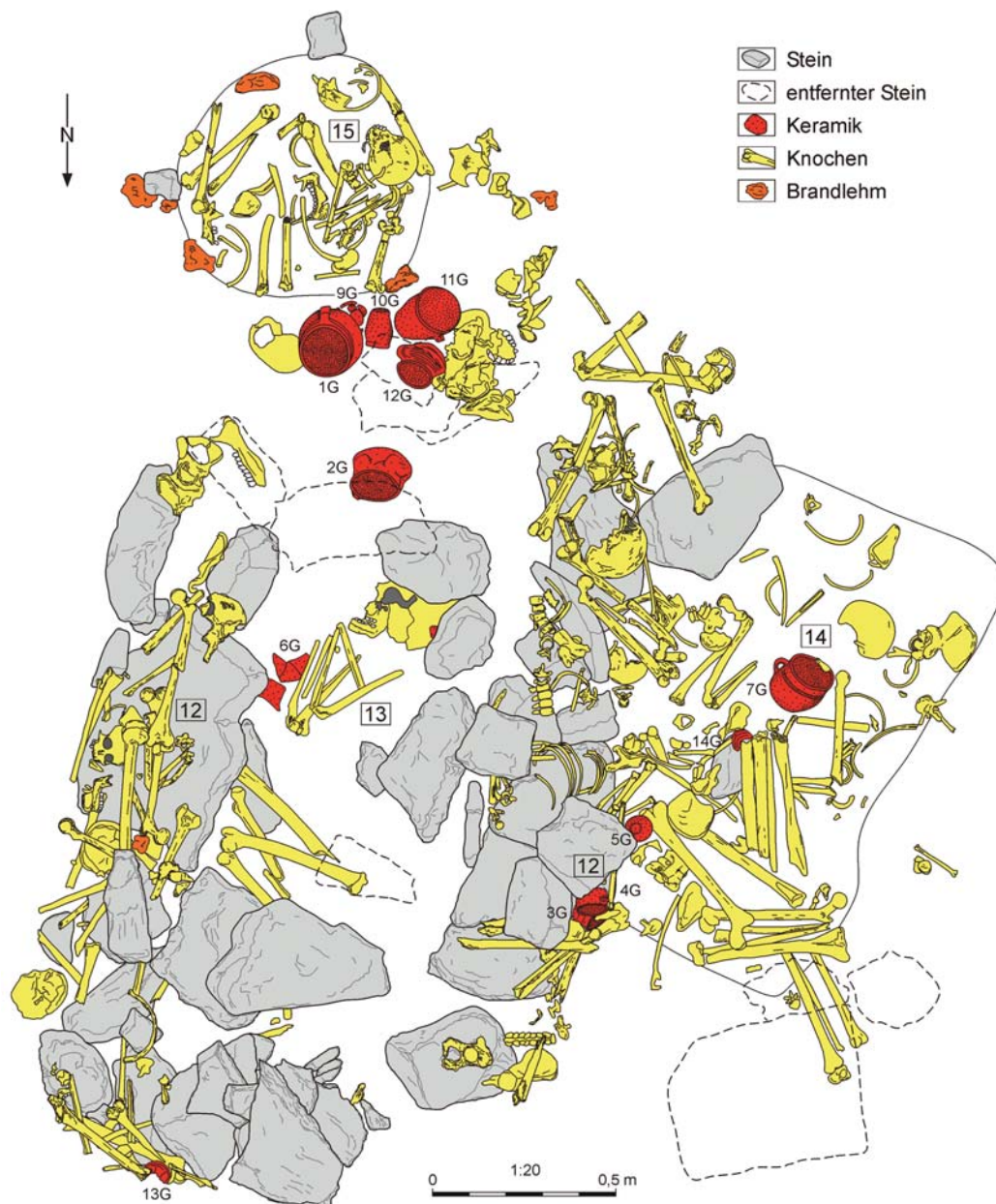
Abb. 11 Watenstedt (Lkr. Helmstedt). Befunde 12-15. Gesamtplan mit mehreren interpolierten Grabungsstadien (gestrichelt: die bereits entfernten Steine mit darunterliegenden Skelettresten und Gefäßen). Zeichnung gedreht und der Ausrichtung von Abb. 3 angepasst. – (Graphik H. Marx).
