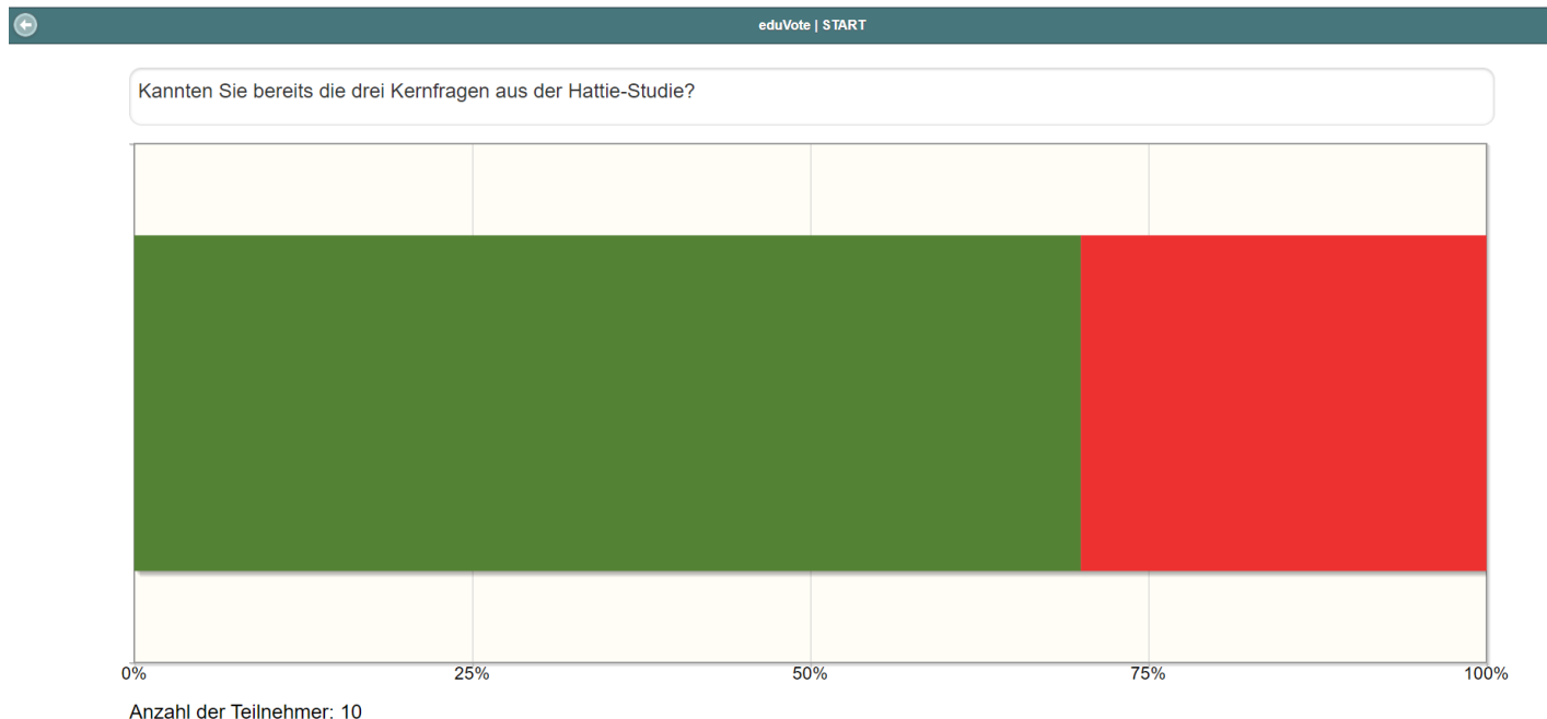
Web-Browser (Chrome)
