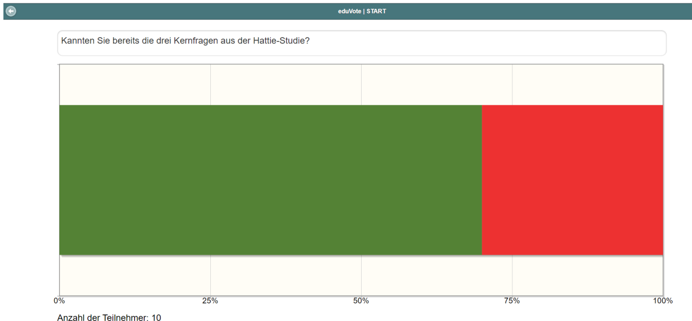
Web-Browser (Chrome)
