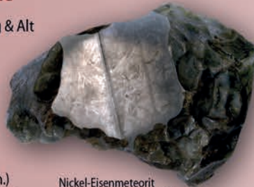
Nickel-Eisenmeteorit Emsland, gefunden 1940
